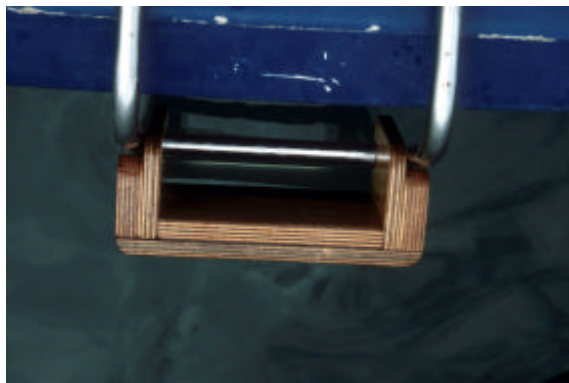
Soporte motor fuera borda para emergencia
